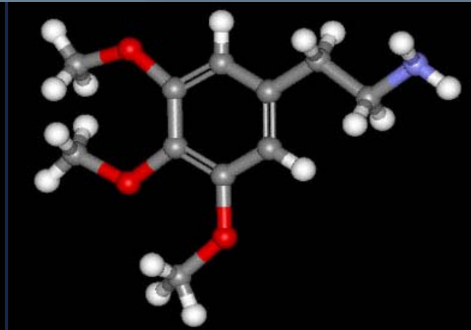
meszkalin
