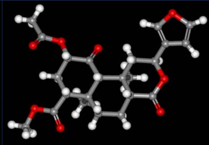
szalvinorin-A
