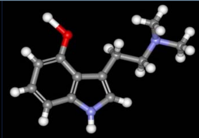
pszilocibin
